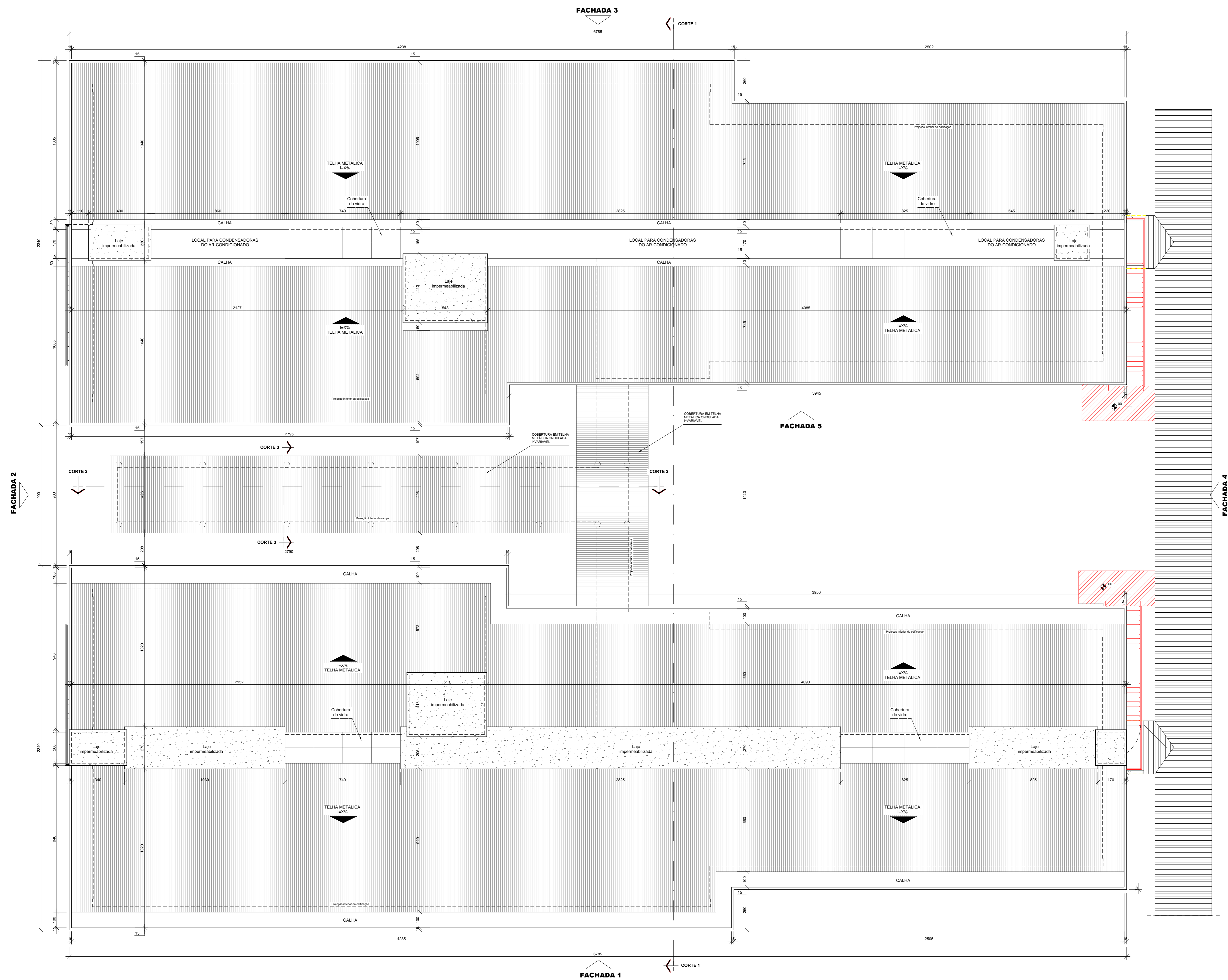
PLANTA DE MODIFICAÇÃO E ANÁLISES CBM-DF - PLANTA DE COBERTURA 1:100
